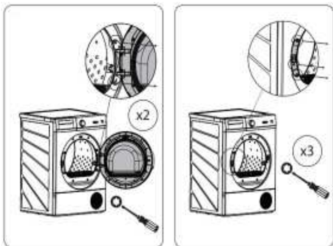
1. Remove door and door hinge
