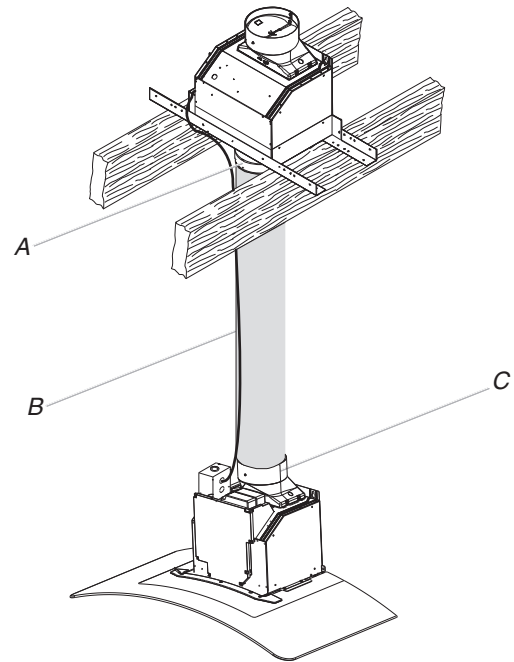
A. Raccord de transition du ventilateur déporté intelligent (en bas) B. Circuit d'évacuation C. Raccord de transition de la hotte
