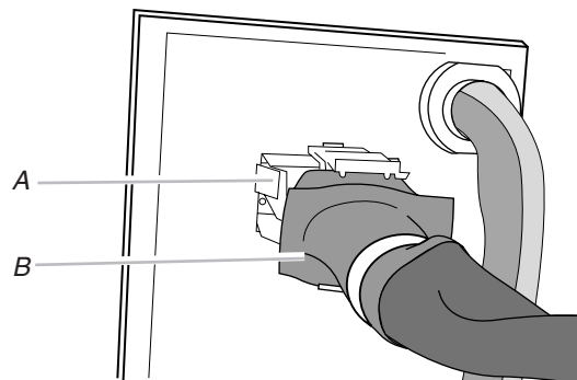
A. Conector de caja de cableado B. Conector de suministro de energía de la campana
