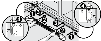
Instalación de la rejilla inferior
