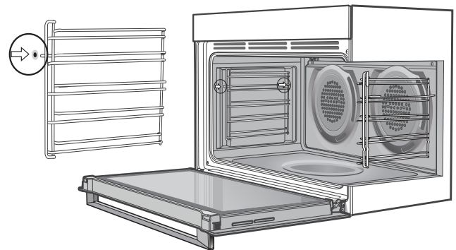
Figure 10: Installation d'une grille latérale Easy Access
