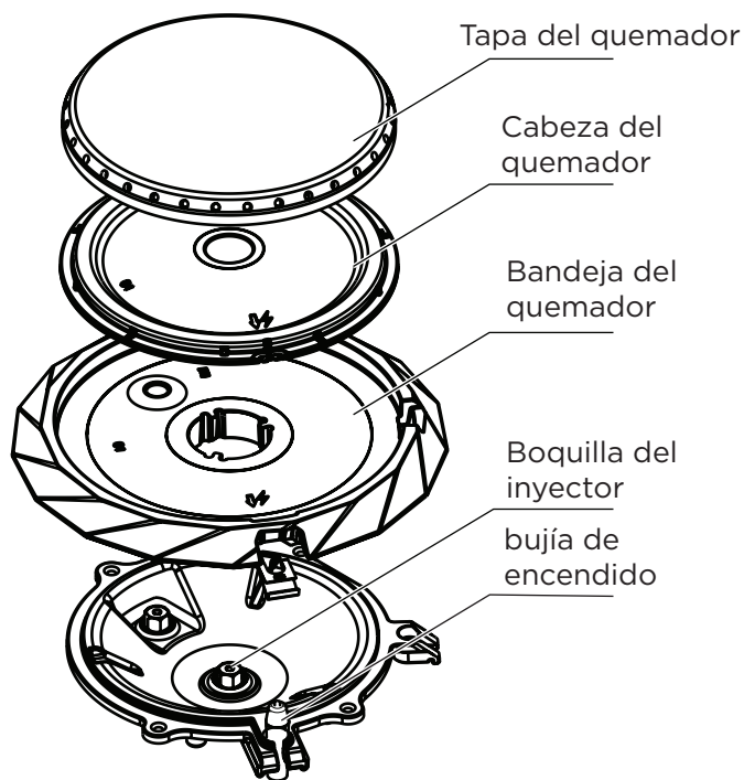
Figura 1: Conjunto De Quemador Doble
