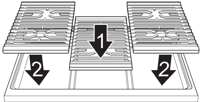
Figura 4: Instale las rejillas
