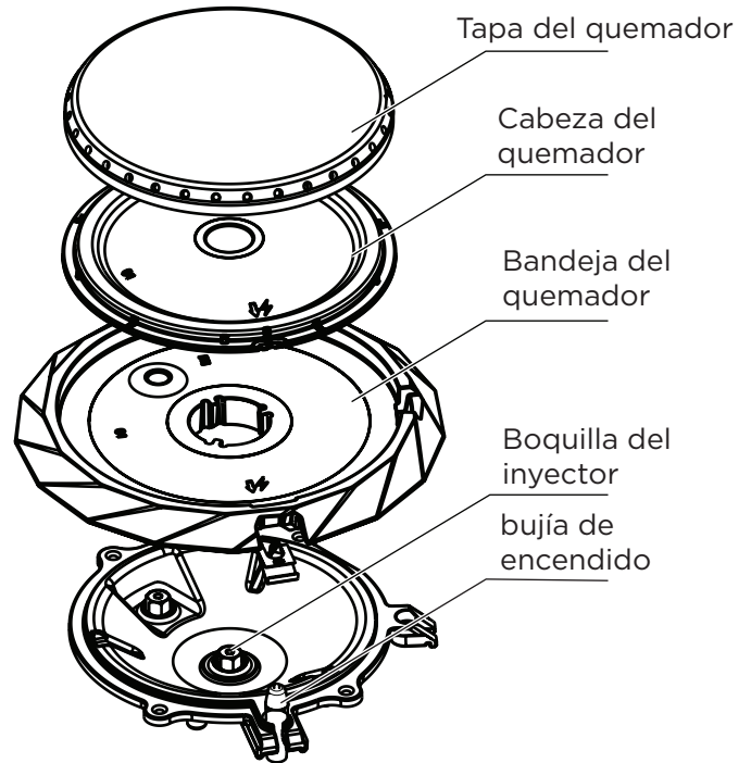
Figura 19: Componentes extraíbles del quemador
