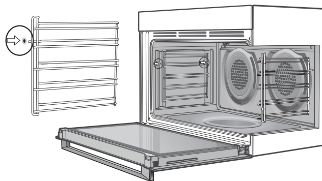
Figura 10: Instalación de soportes laterales de fácil acceso
