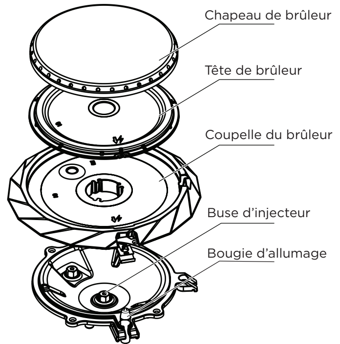
Figure 1: Ensemble Double Brûleur
