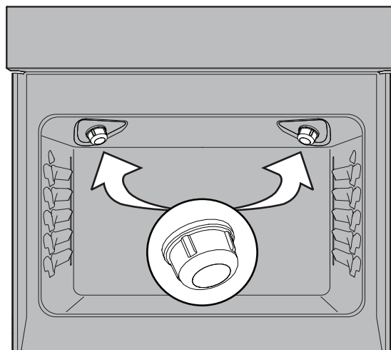
Figure 10: Lumière halogène du four encastré
