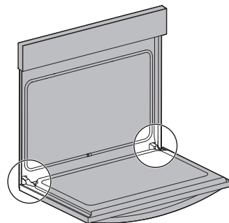
Figure 19: Emplacement de la charnière de la porte
