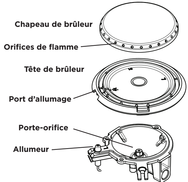
Figure 17: Chapeau de brûleur, tête de brûleur, allumeur et orifice
