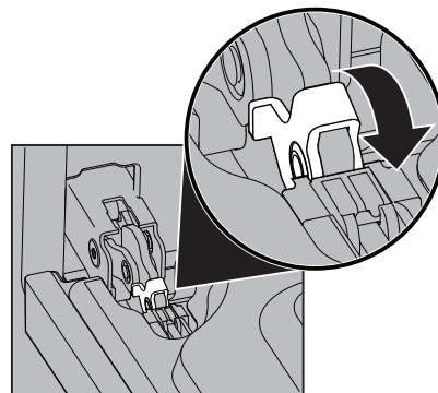
Figure 20: Serrure de charnière de porte
