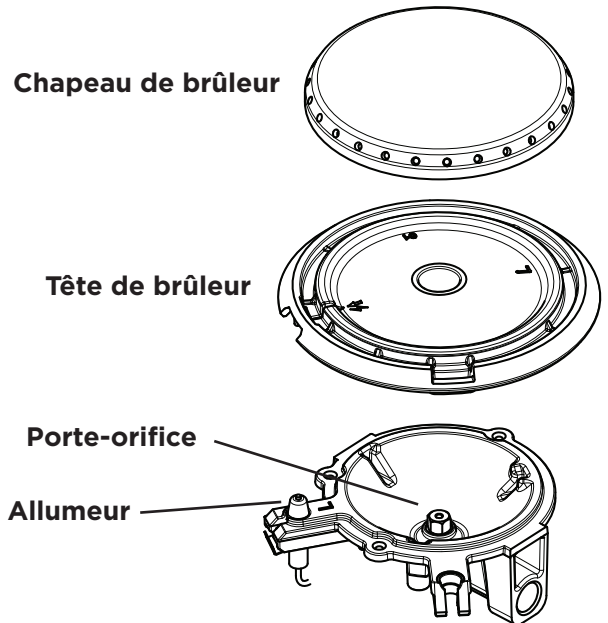
Figure 14: Chapeau de brûleur, tête de brûleur, allumeur et orifice
