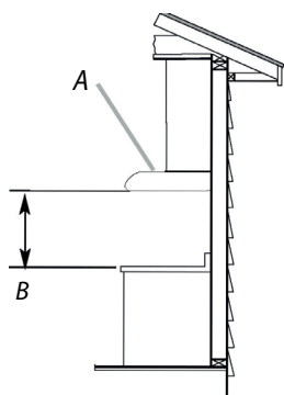
Recirculation
