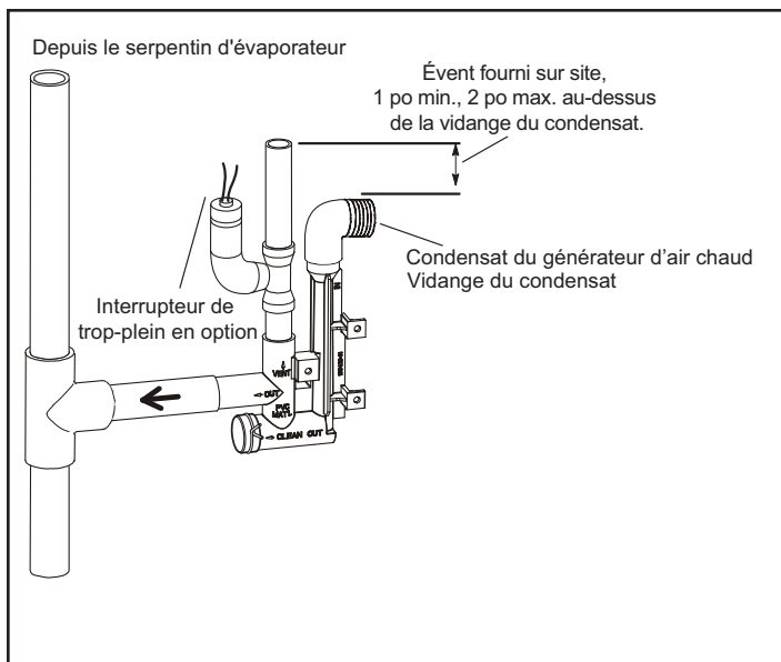
Figure 43. Purgeur de condensat avec interrupteur de trop-plein
