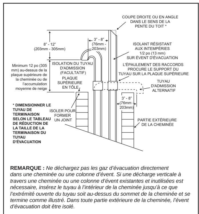
Figure 32. Application de ventilation directe avec une cheminée existante
