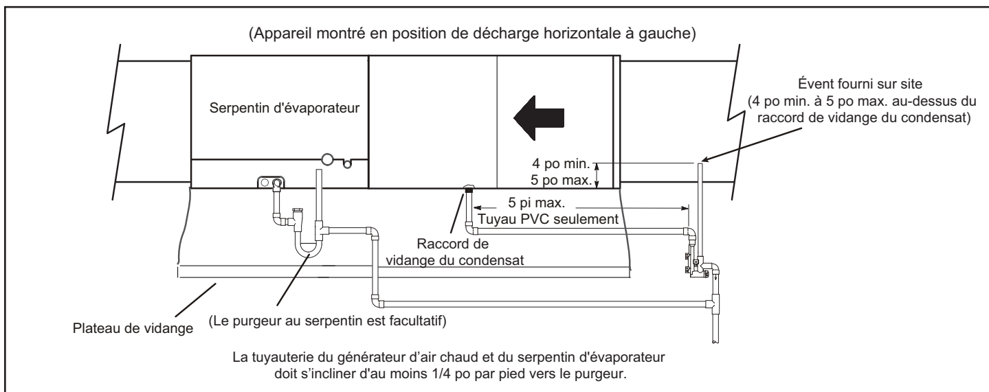
Figure 41. Générateur d'air chaud avec serpentin d'évaporateur utilisant un drain commun
