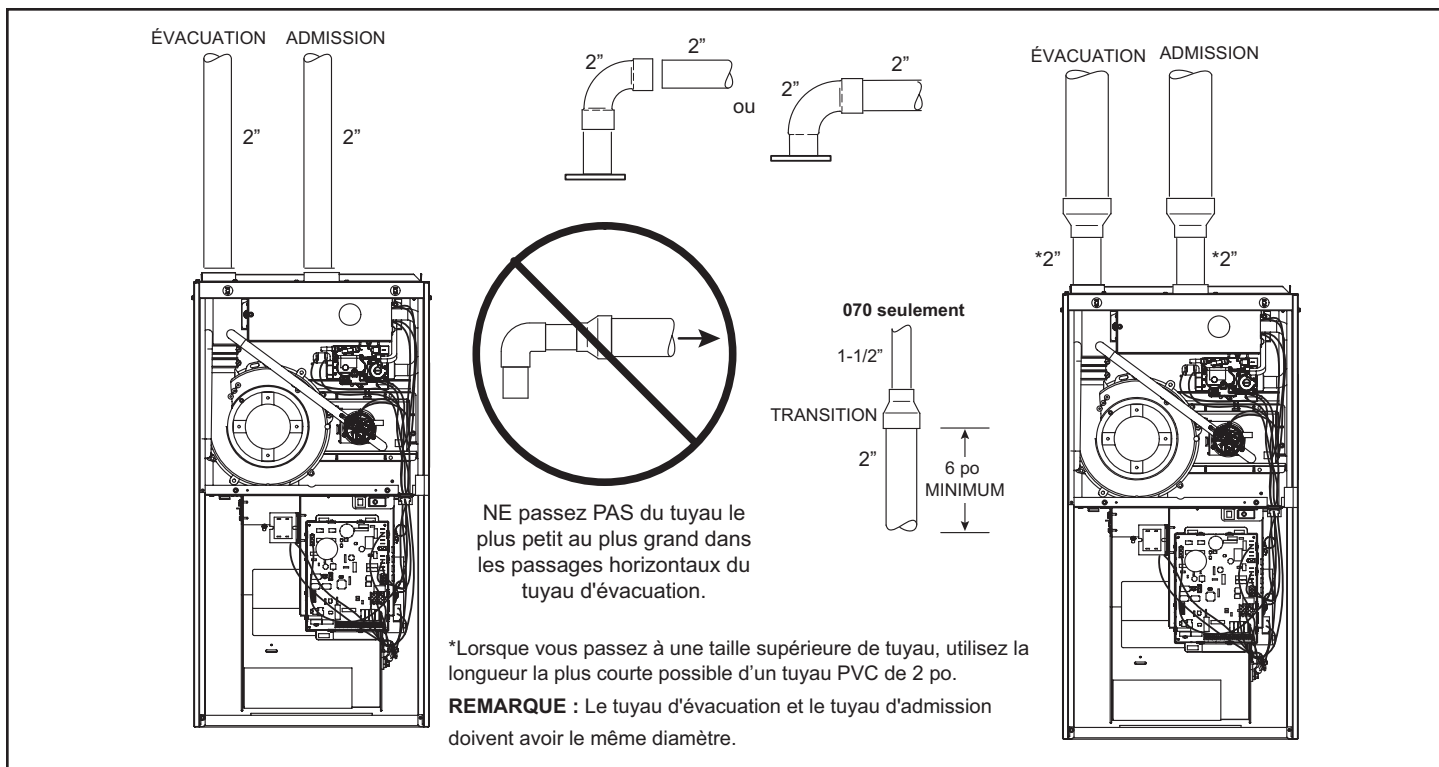
Figure 21. Installation typique des raccords de tuyaux d'évacuation et d'admission et du purgeur de condensat dans l'application à ventilation ascendante
