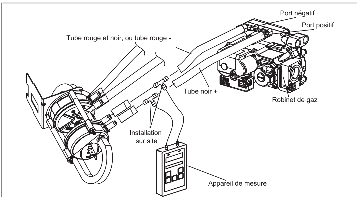
Figure 49. Mesure du signal de fonctionnement (Delta P)
