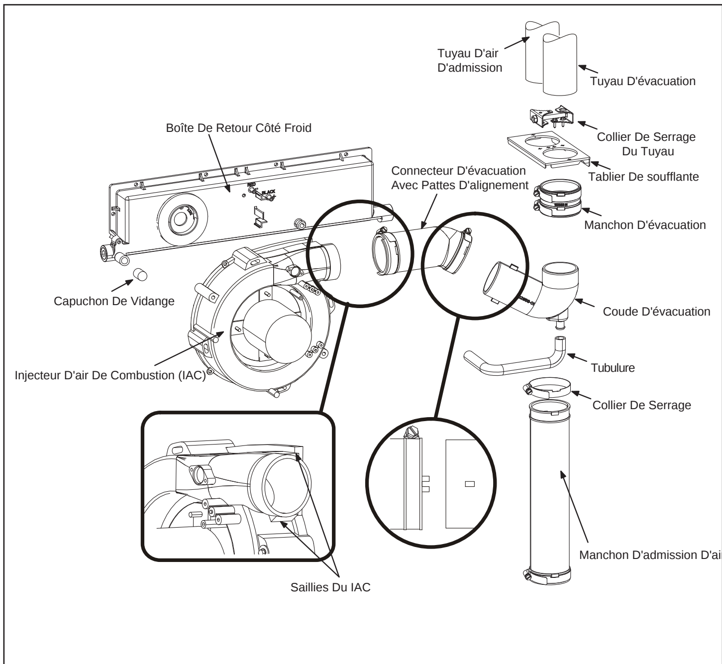
Figure 19. Assemblage injecteur d'air de combustion / boîte de tête côté froid / tuyau d'évent
