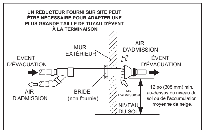
Figure 33. Terminaison murale concentrique à ventilation directe 71M80, 69M29 OU 60L46 (É.-U.) 44W92 ou 44W93 (Canada)
