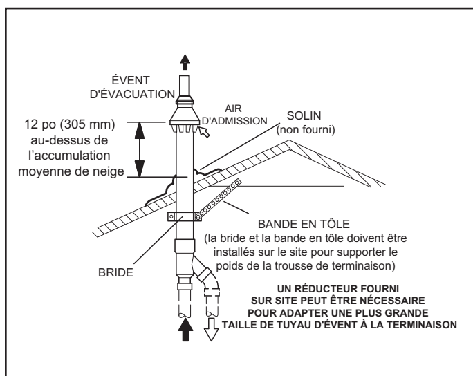
Figure 31. Terminaison de toit concentrique à ventilation directe 71M80, 69M29 OU 60L46 (É.-U.) 44W92 ou 44W93 (Canada)
