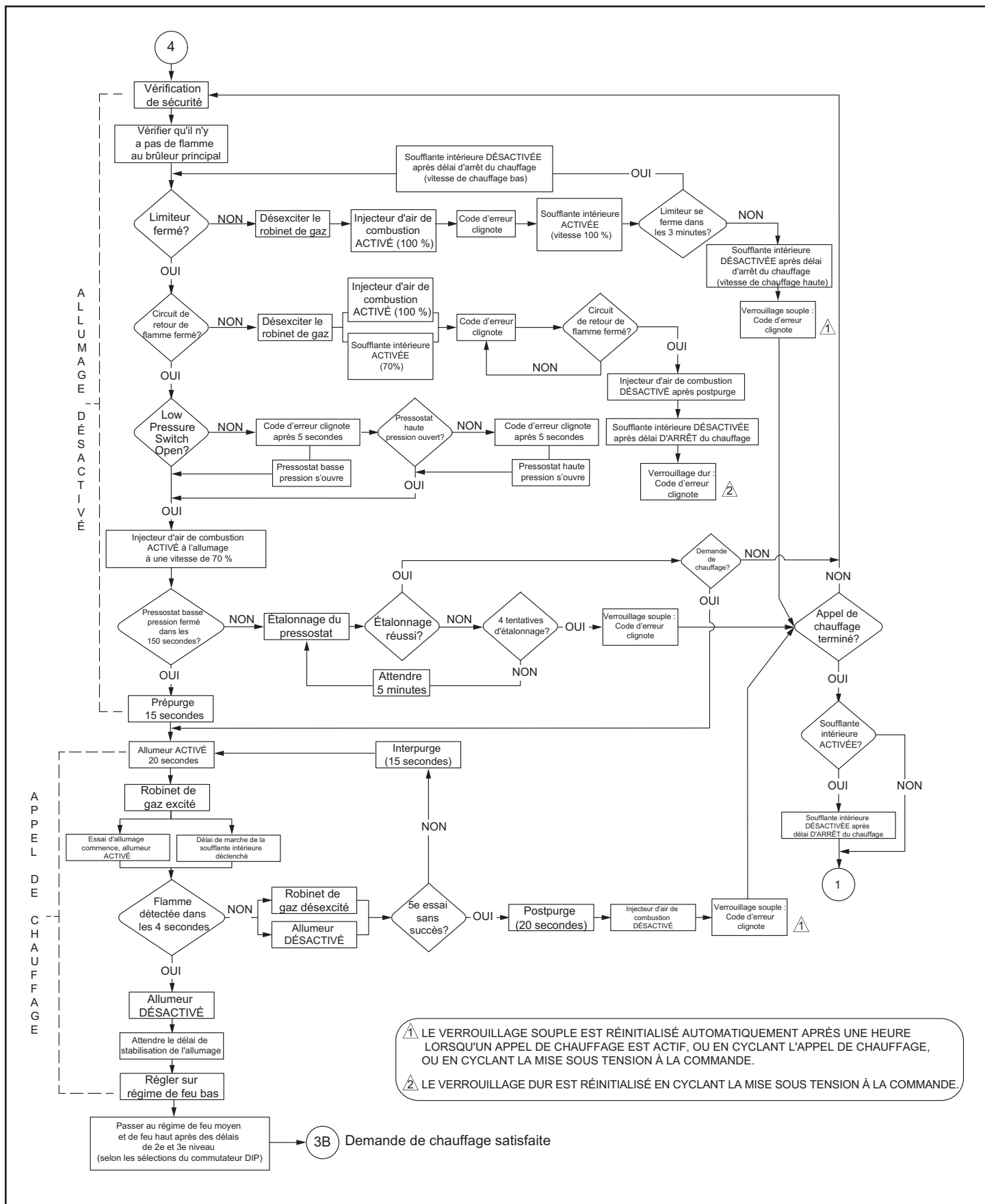
Figure 57. Allumage et appel de feu bas avec un thermostat à un niveau
