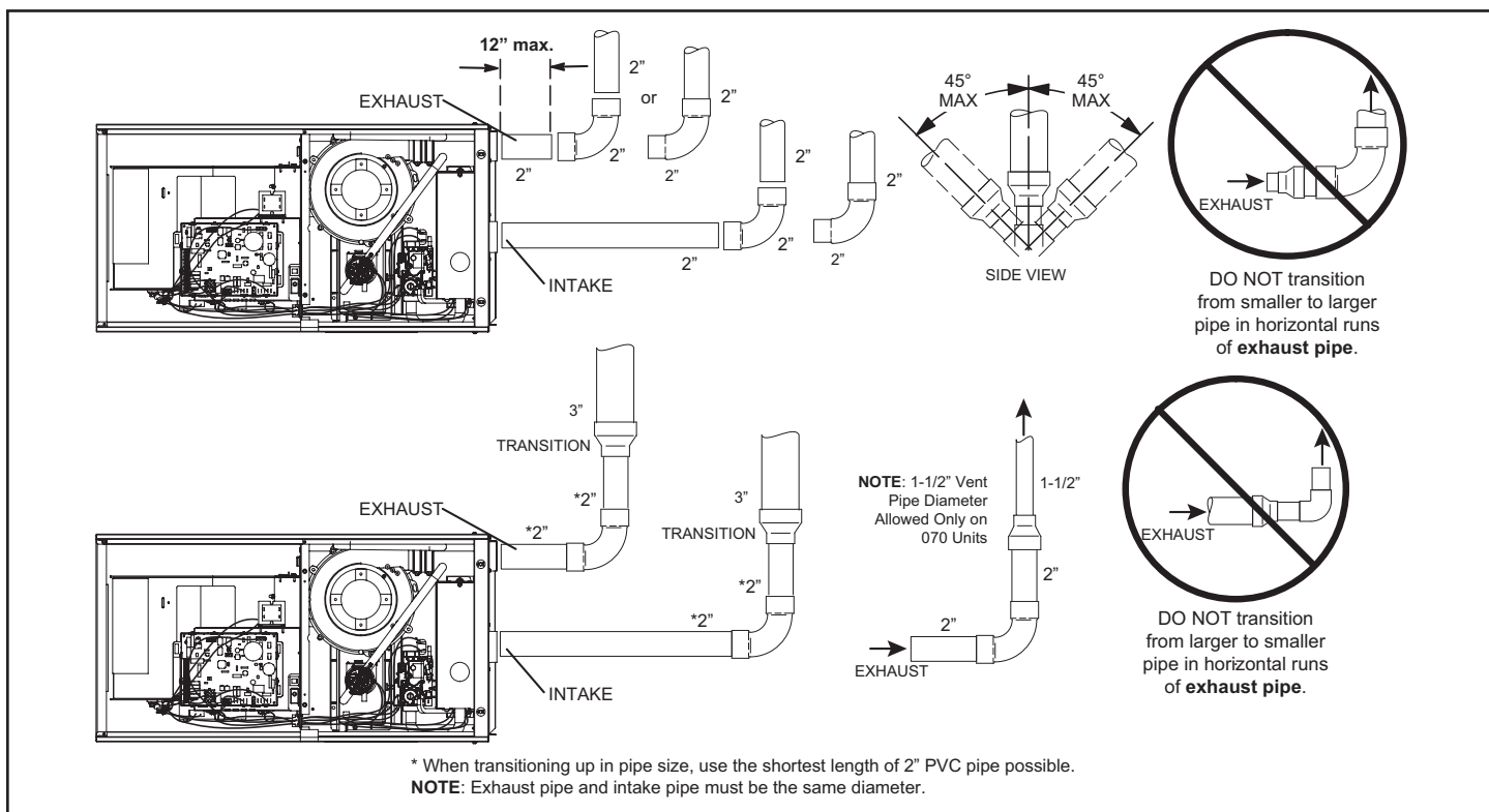
Figure 22. Installation typique des raccords des tuyaux d'évacuation et d'admission et du purgeur de condensat dans les applications à ventilation horizontale (décharge à droite illustrée)
