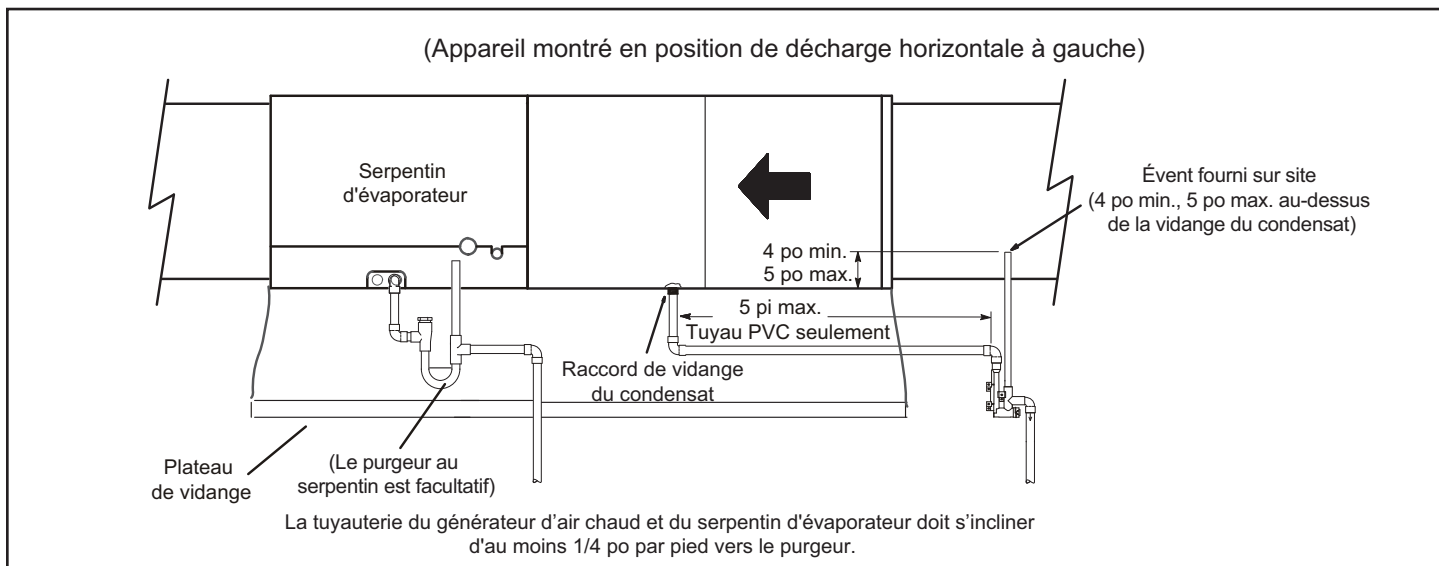
Figure 38. Générateur d'air chaud avec serpentin d'évaporateur utilisant un drain séparé
