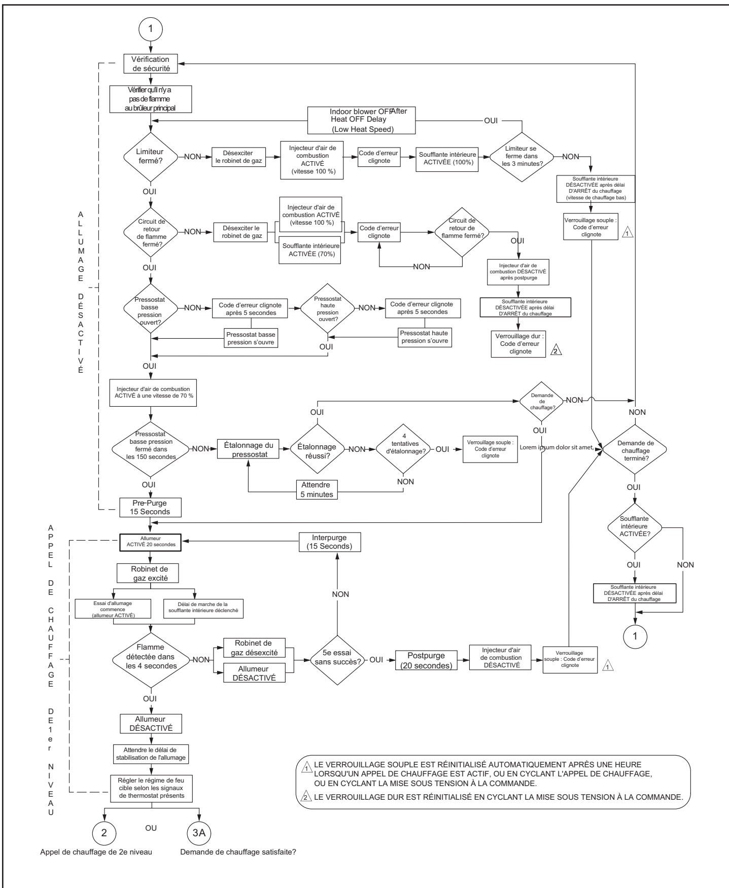
Figure 54. Allumage et appel de feu bas avec un thermostat à deux niveaux
