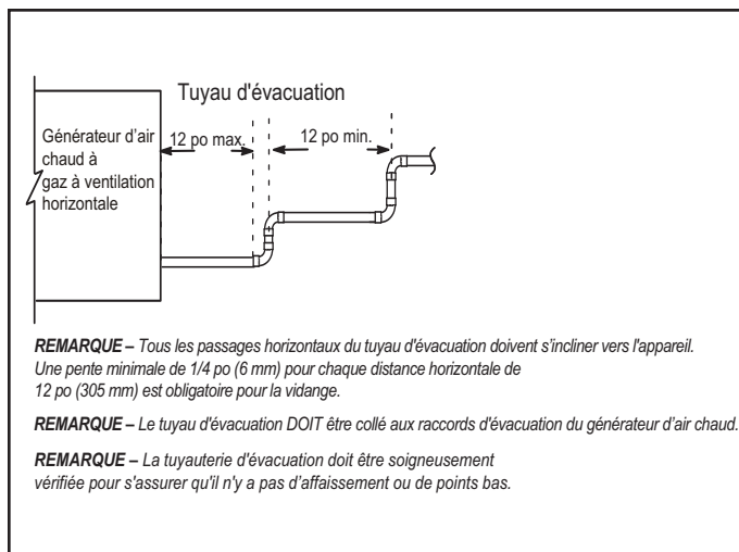
Figure 23. Exigences De Décalage Pour Une Installation Horizontale
