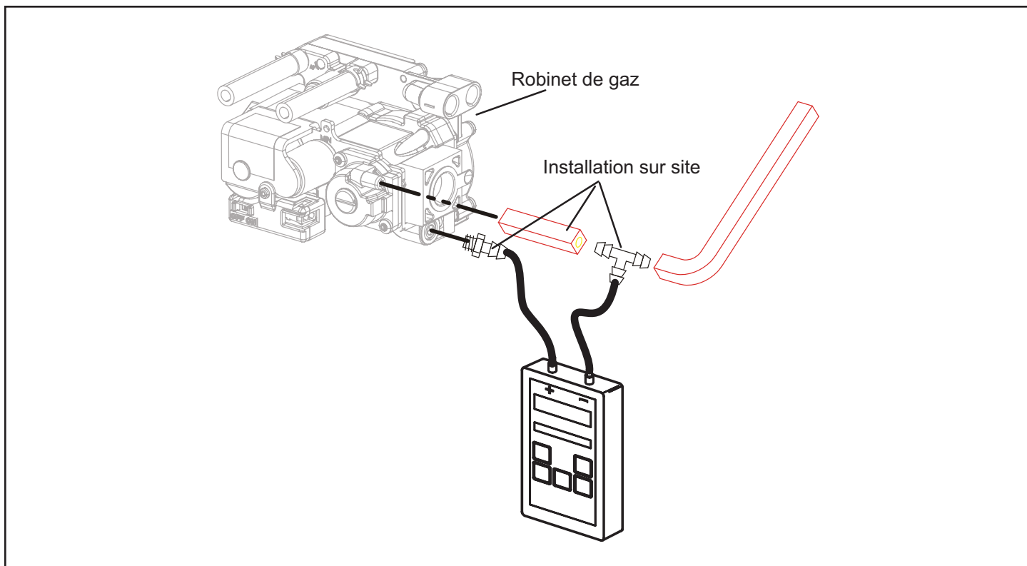
Figure 48. Mesure de la pression du collecteur
