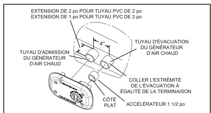
Figure 34. Terminaison de mur latéral à montage affleurant 51W11
