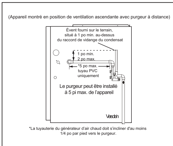
Figure 37. Emplacements du purgeur de condensat
