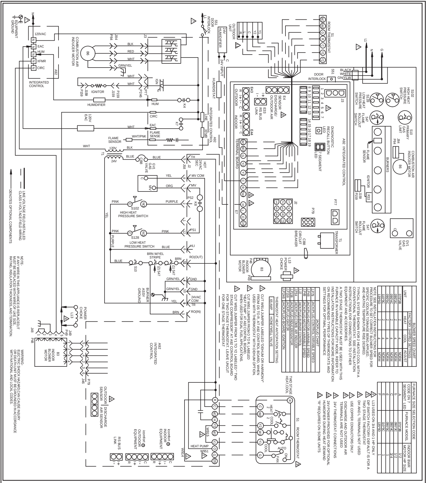
Figure 52. Câblage sur site typique
