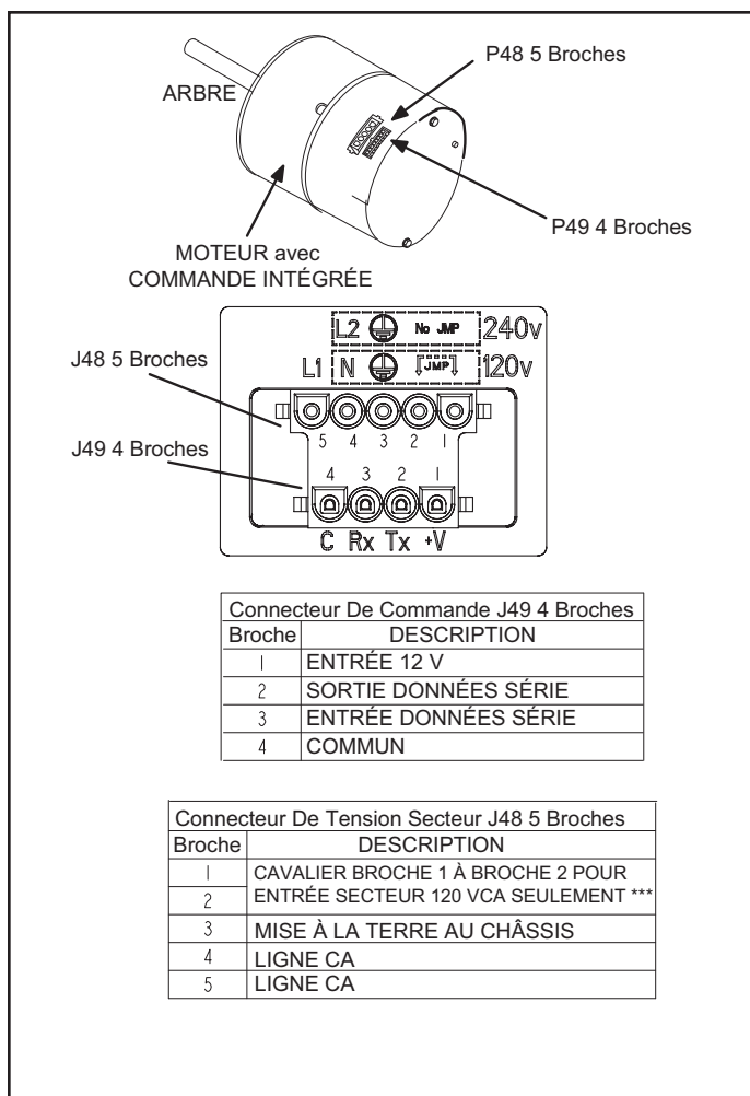
Figure 9. Connecteurs du faisceau B3 de la soufflante
