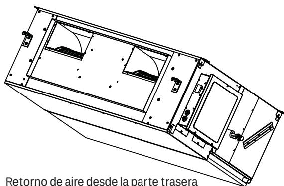
Retorno de aire desde la parte trasera
