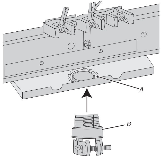
A. Tuerca de retención removible B. Conductor
