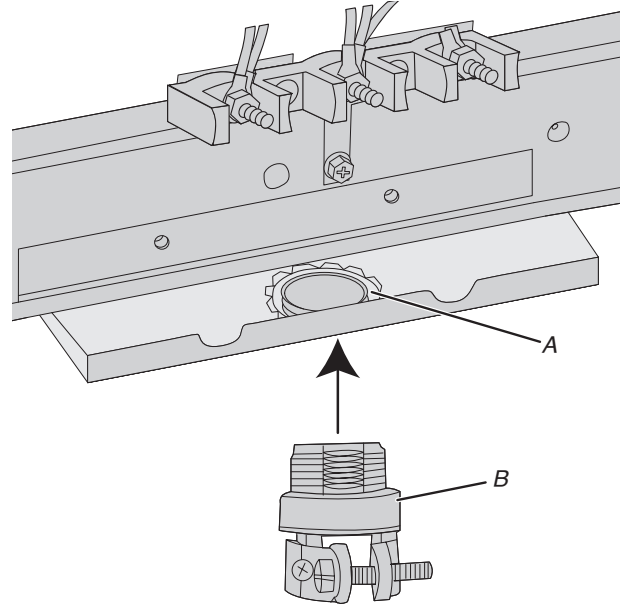
A. Écrou de retenue amovible B. Conduit
