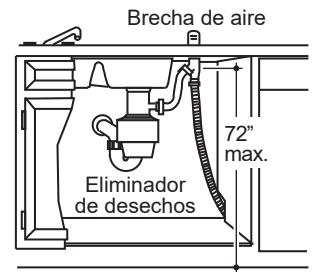
Instalación del eliminador de desechos con brecha de aire
