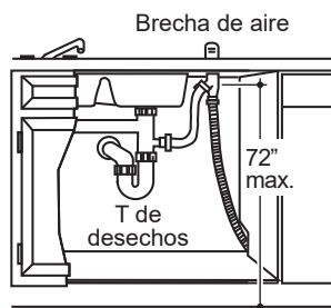
Instalación del T de desechos con brecha de aire
