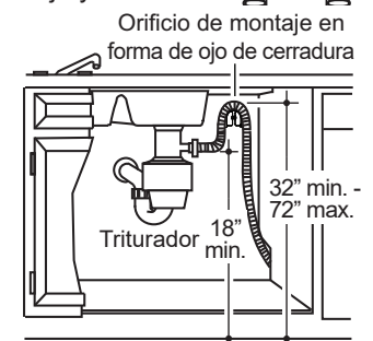
Instalación del triturador con bucle de drenaje alto en el soporte
