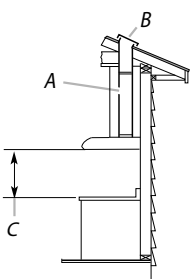
Ventilación a través del techo
