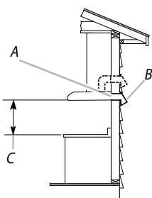
Ventilación a través de la pared
