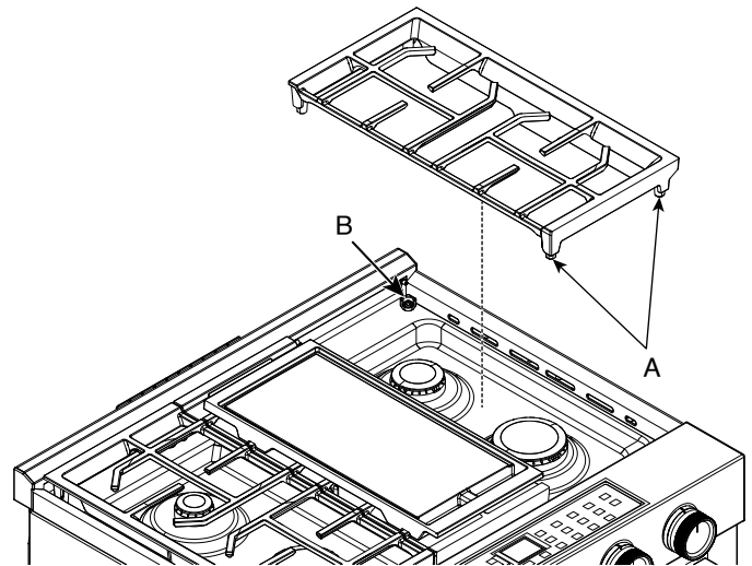
A. Butoir B. Indentations d'alignement
