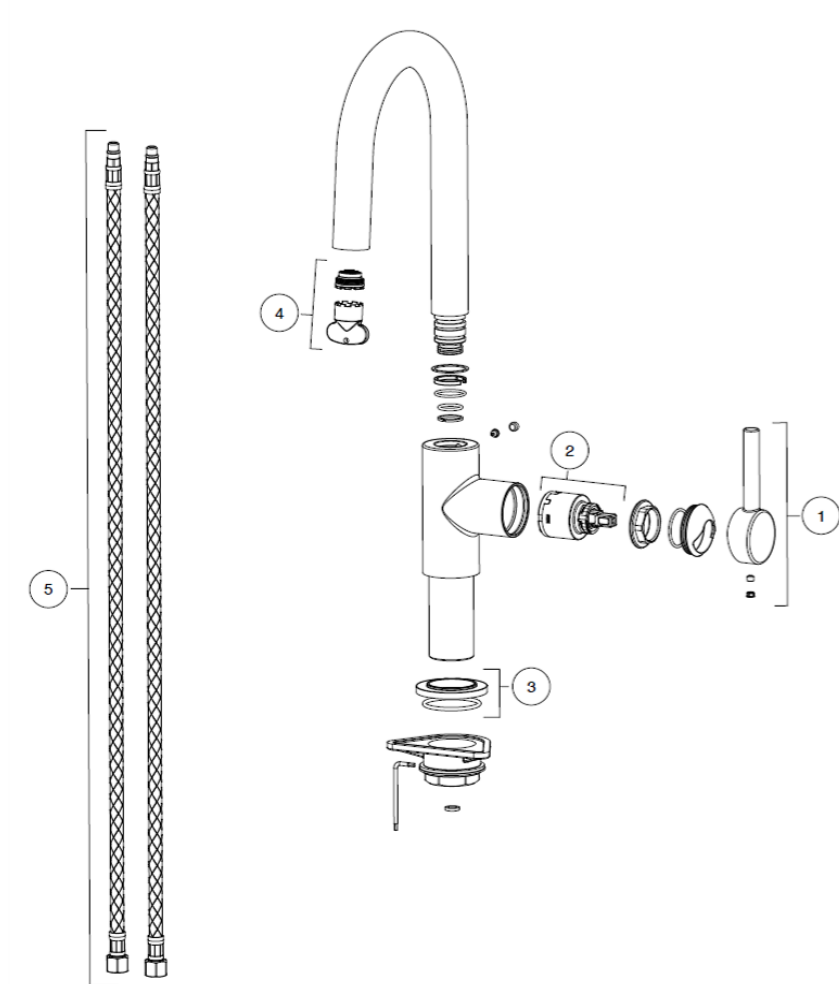
Tap Maris Lario J Bar Swivel SN
